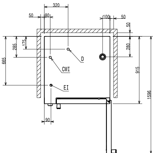
Felülnézet
